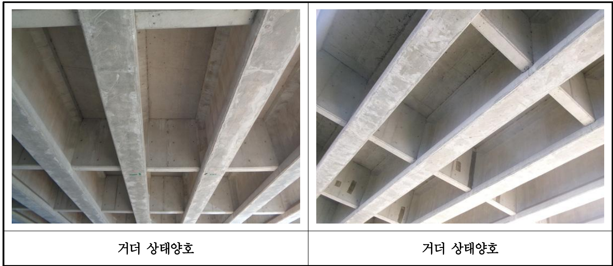
【사진 2.3.5】 거더 손상현황
