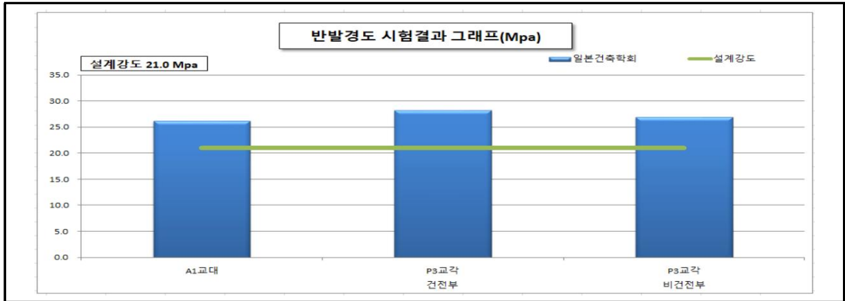
【그림 2.4.4】 반발경도시험(하부구조)
