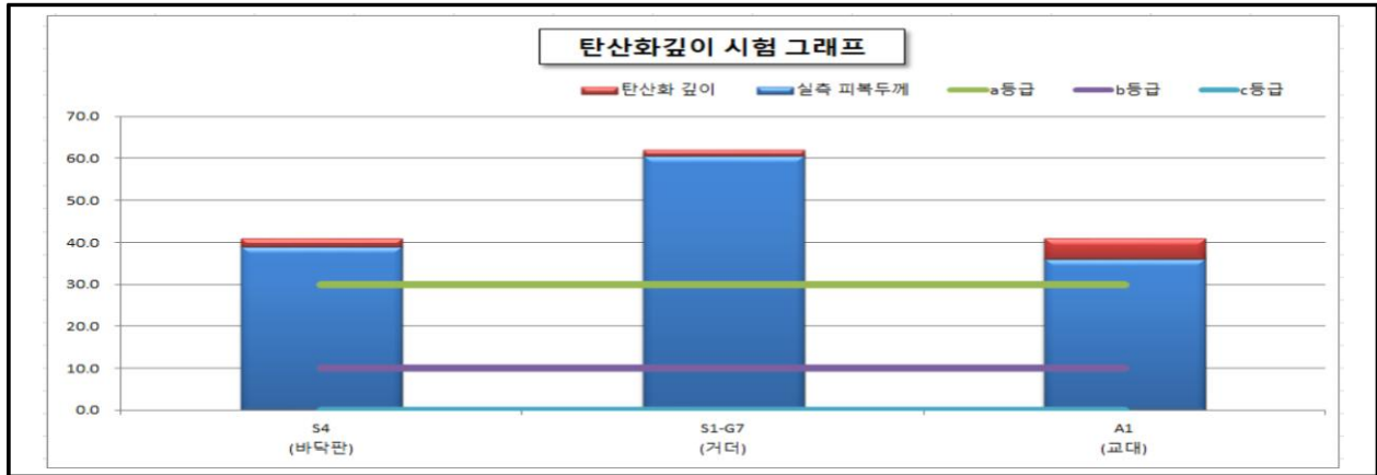
【그림 2.4.5】 탄산화깊이 시험 그래프
