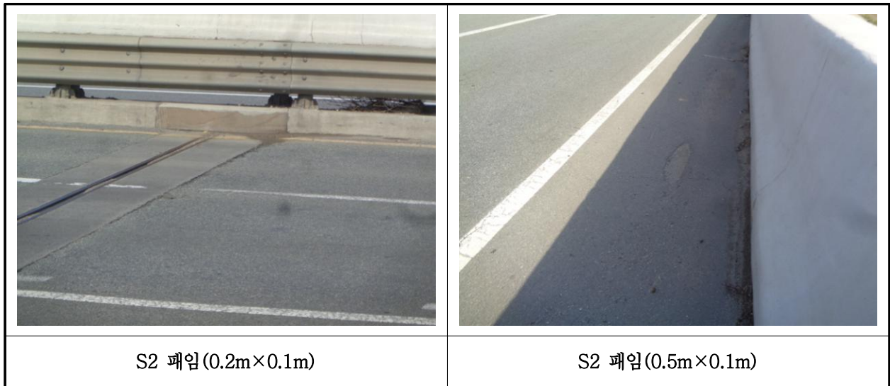
【사진 2.3.20】 교면포장 손상현황
