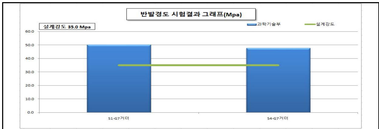
【그림 2.4.3】반발경도시험(상부구조 교강도)
