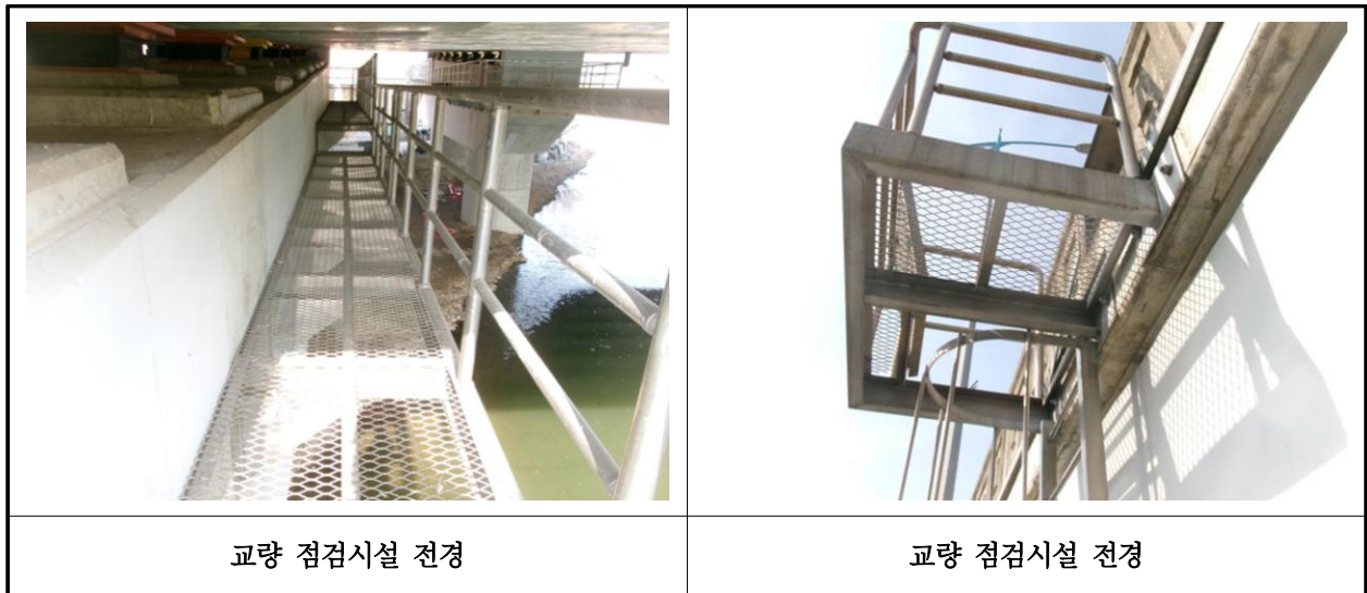
【사진 2.3.26】 교량 점검시설 손상현황
