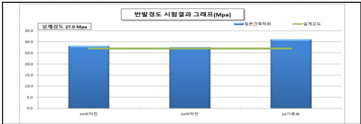
【그림 2.4.2】반발경도시험(상부구조)
